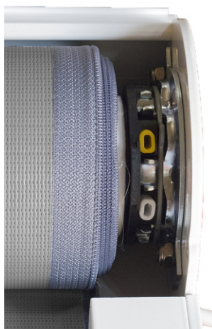
Coffre Zip à moteur et bandes latérales Zip
